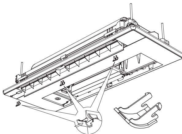
Painel com parafusos embutidos
